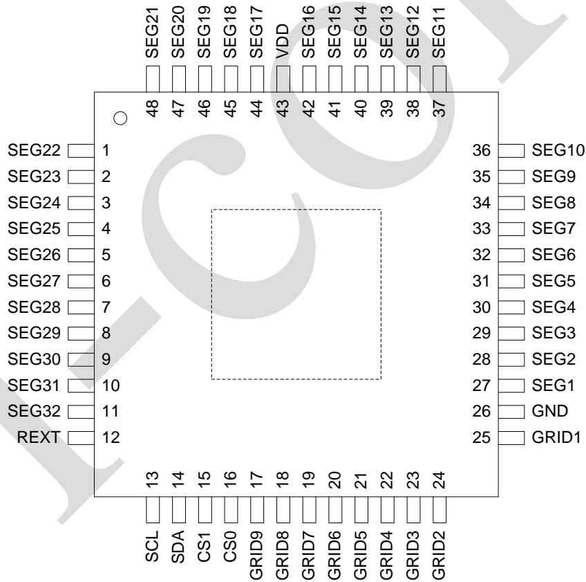
ELQFP48/ETQFP48
