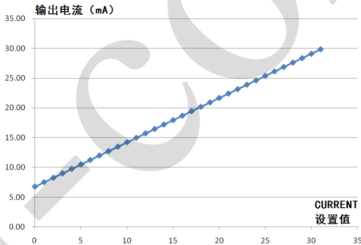
图 4 CURRENT 设置与 SEG 输出电流关系
